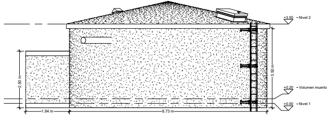
① Vista - Norte 1 : 50
