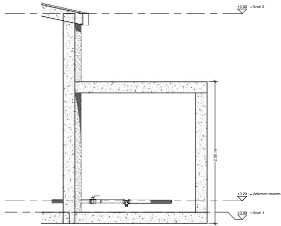
③ Cuarto de Máquinas 1 : 20
